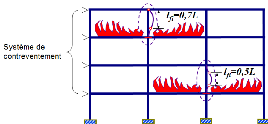
Longueurs de flambement en situation d'incendie de poteaux d'ossatures contreventées
